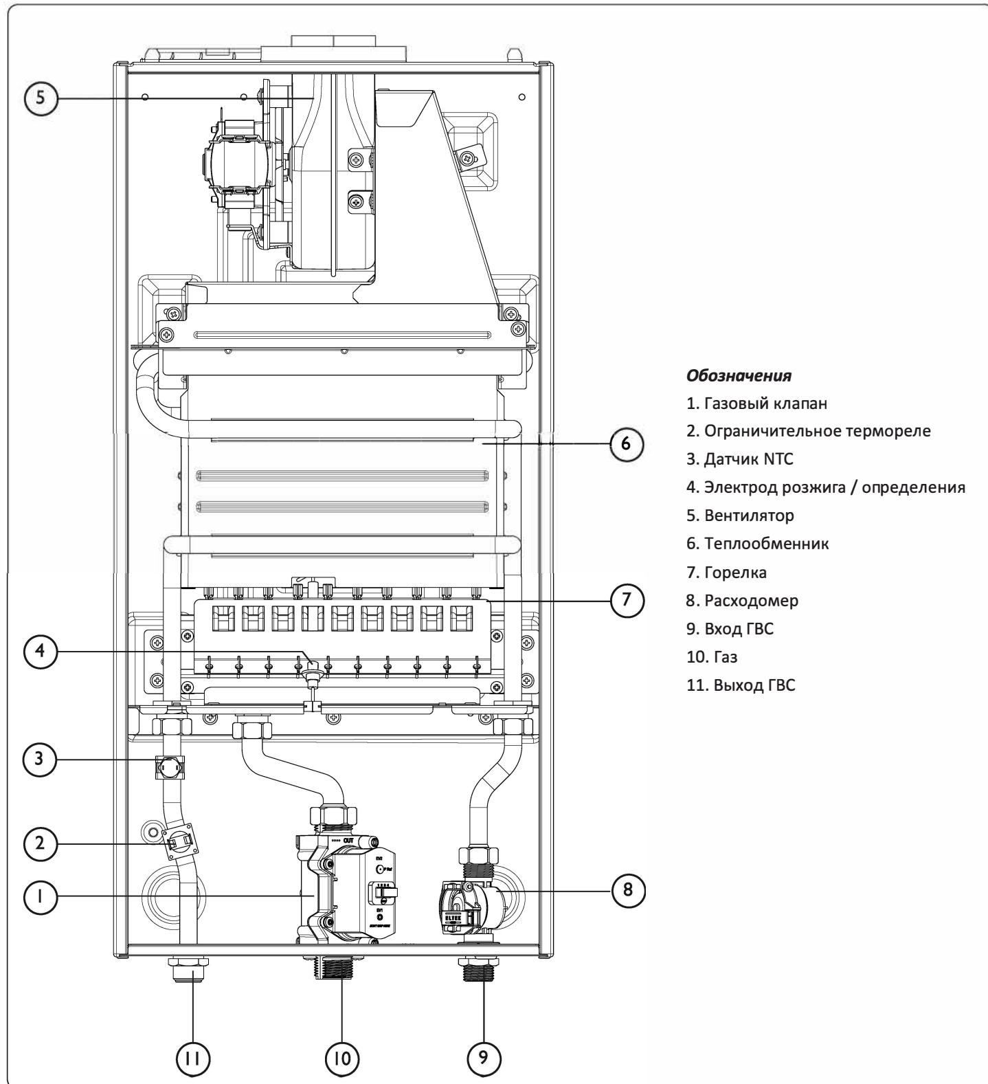
Рис. 1 – Компоненты водонагревателя
