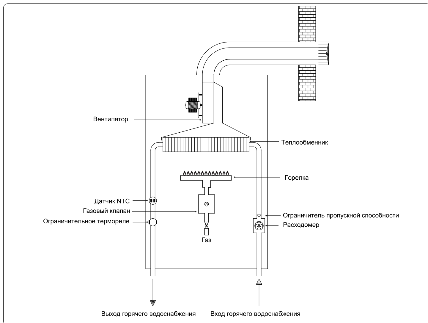
Рис. 3 – Гидравлическая сеть
