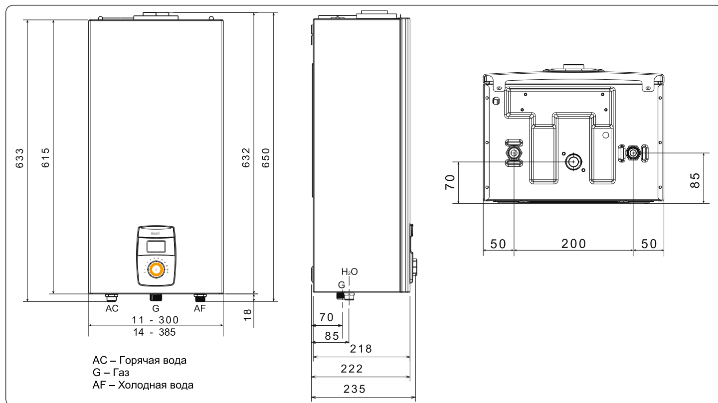
Рис. 2 – Монтажный размер – Измерения в мм
