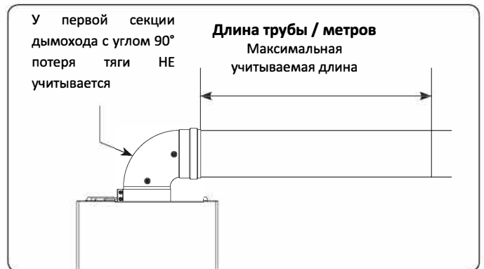
Рис. 10 – Максимальная длина трубы (см. следующую таблицу)
