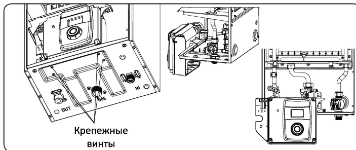
Рис. 17 – Снятие вентилятора
